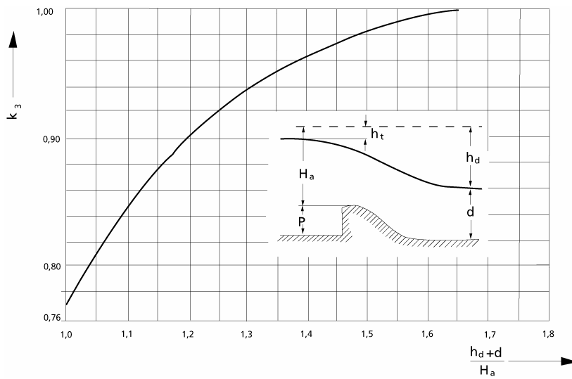
Figur 3-5. Overløpskoeffisiensens avhengighet av nedstrøms bunn-nivå. h_d = hastighetshøyden, d = vann dybden
