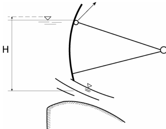
Figur 3-8 Underløpsluke
