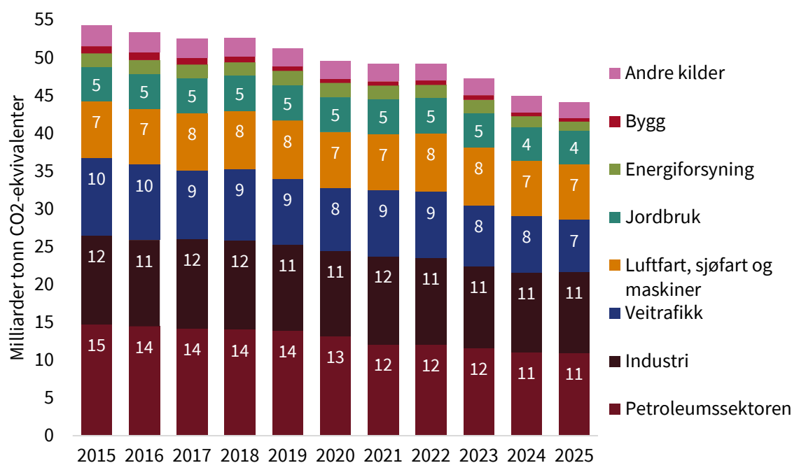
Figur 1-5 Utslipp av klimagasser i Norge etter sektor fra 2015 til 2025. Kilde: SSB.
