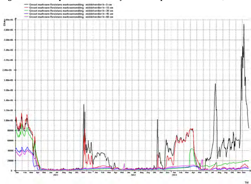
Figur 14. Resistansmålinger ved ulike dybder målt i perioden 2011-2013;
