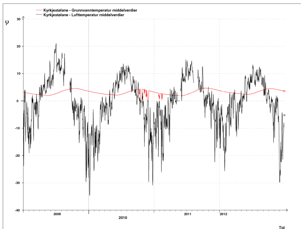
Figur 6. Grunnvanns- og lufttemperatur målt i 2009-2012
