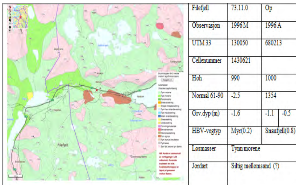
Figur 1. Oversikt over Filefjell målestasjon.
