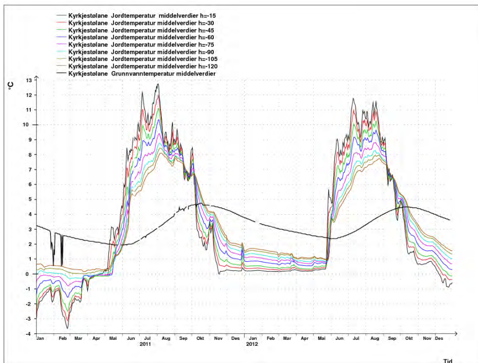
Figur 8. Grunnvann-, og jordtemperaturer 2011-2012.
