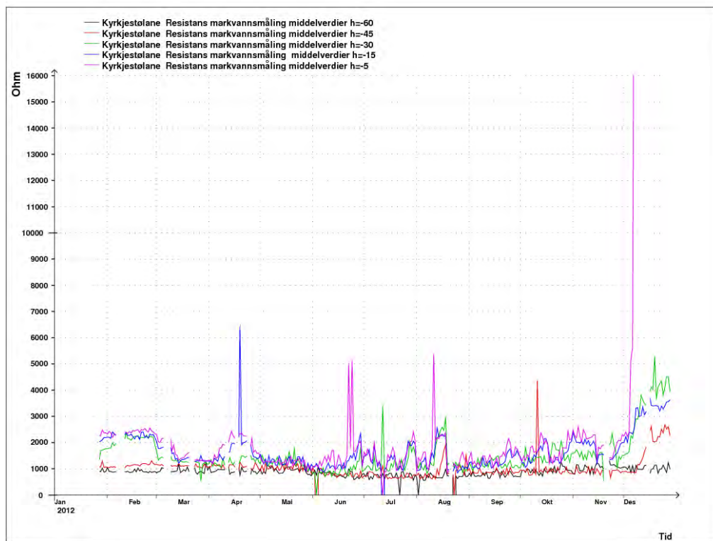
Figur 7. Resistansmålinger ved forskjellig dyp (cm) for Filefjell 2012 (dataene er ukontrollert).
