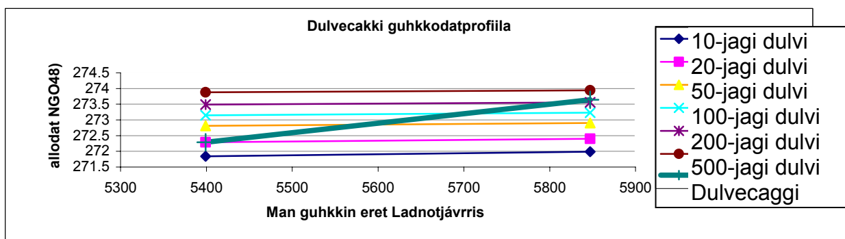
Sárggastus 4.3 Dulvecakki guhkkodatprofiila iešguđet dulvviin
