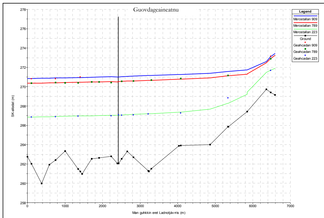
Sárggastus 3.1 Meroštallojuvvon ja geahčaduvvon čáhcedásit Guovdageaineanus Máze bokte
