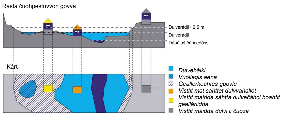
Sárggastus 4.1 Prinsihppasárggastus mii čájeha vuollegis eatnamiid čuoggáid ja geallerkeahtes guovllu
