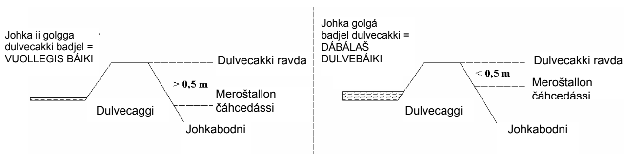
Sárggastus 4.2 Prinsihppasárggastus mii čájeha dulvecakki ja sihkarvuodaráji
