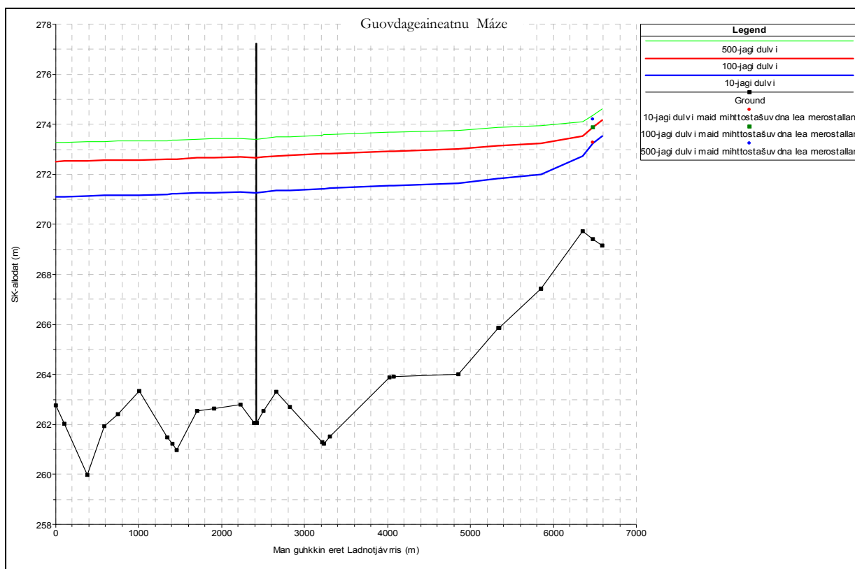
Sárggastus 3.2 Meroštallojuvvon čáhcedásiid guhkkodatprofiilla 10-100 ja 500-jagi dulvviin
