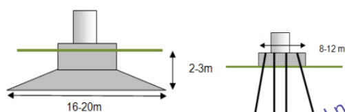
Figur 2-2: Illustrasjon av gravitasjonsfundament (til venstre) og forankringsfundament (til høyre)
