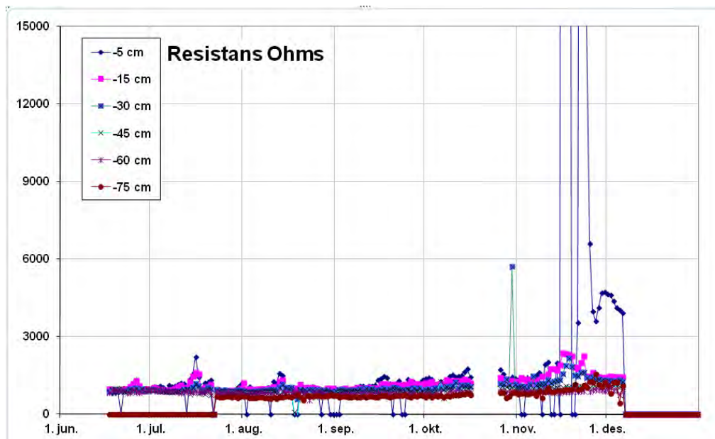
Figur 7. Restistansmålinger for Filefjell 2011.
