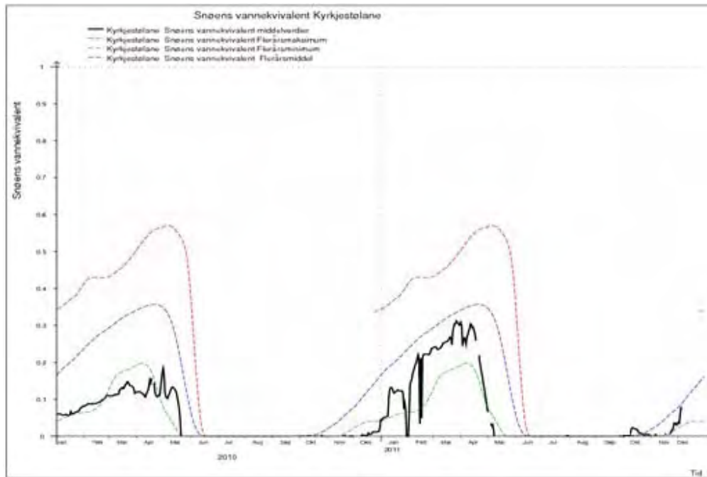
Figur 5. Snøens vannekvivalent målt i 2010-2011 sammenlignet med flereårsmiddel, største og minste observerte snøens vannekvivalent (stiplet) for perioden 1968-1997 (minus årene i perioden 1976-1979, 1989-1993).
