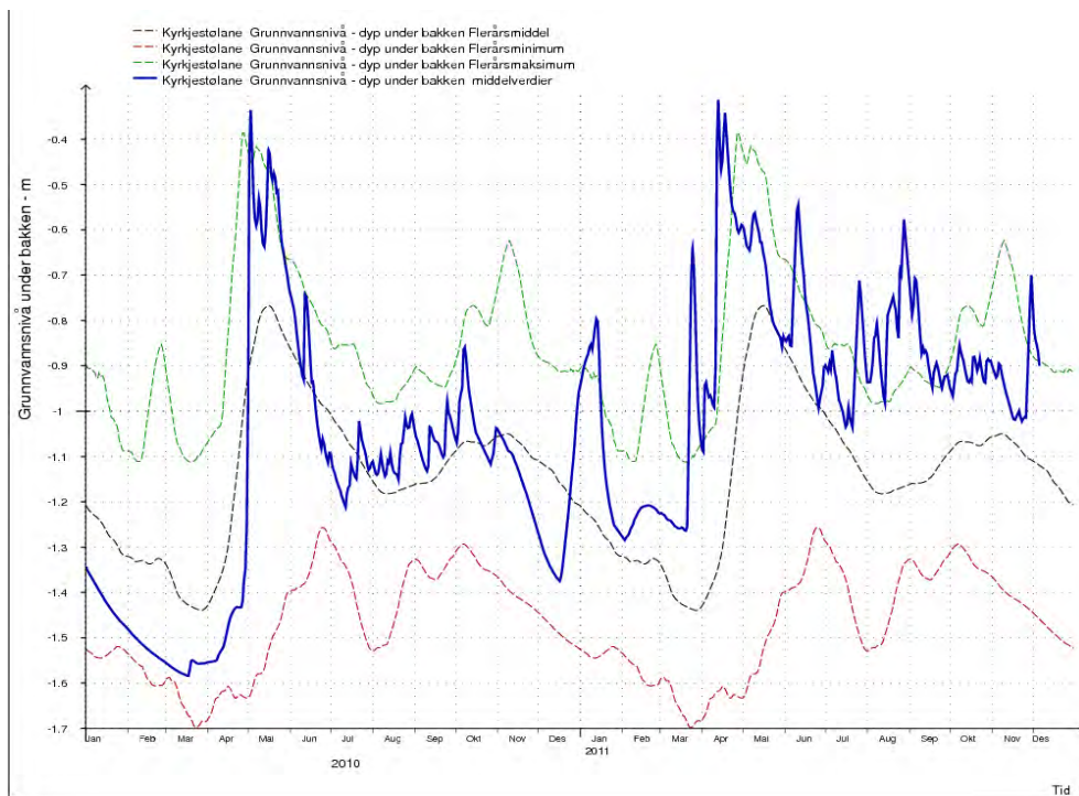
Figur 4. Grunnvannsstand i 2010-2011 (uthevet) sammenlignet med middel, største og minste observerte grunnvannsstand (stiplet) 9 , for perioden 1997-2007 i rør-Kyrkjestølane (interpolasjon på 100 dager).
