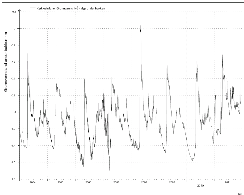
Figur 3. Observerte grunnvannsstand i rør-Kyrkjestølane i perioden 2004-2011;
