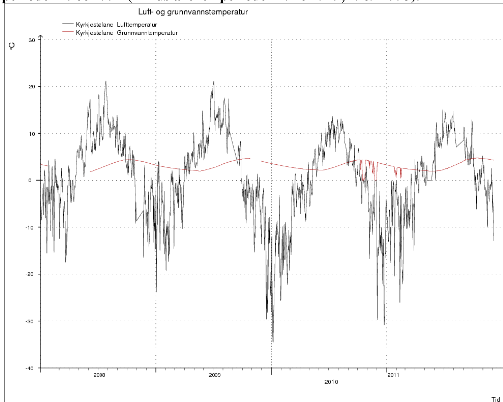
Figur 6. Grunnvanns- og lufttemperatur målt i 2008-2011
