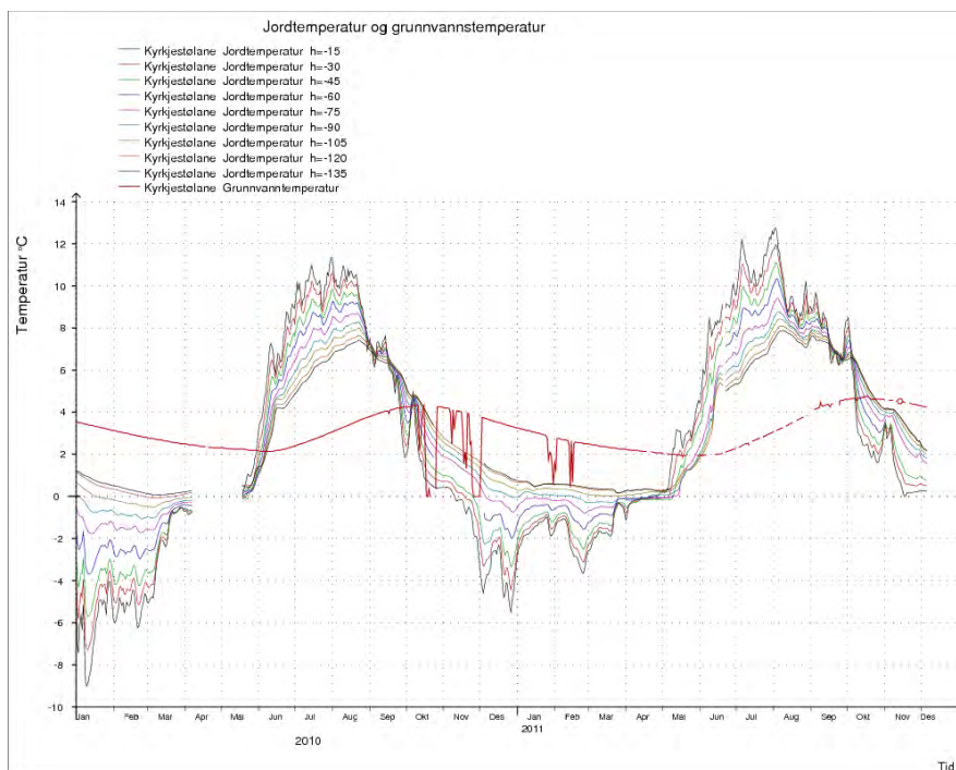
Figur 8. Grunnvann-, og jordtemperaturer 2010-2011
