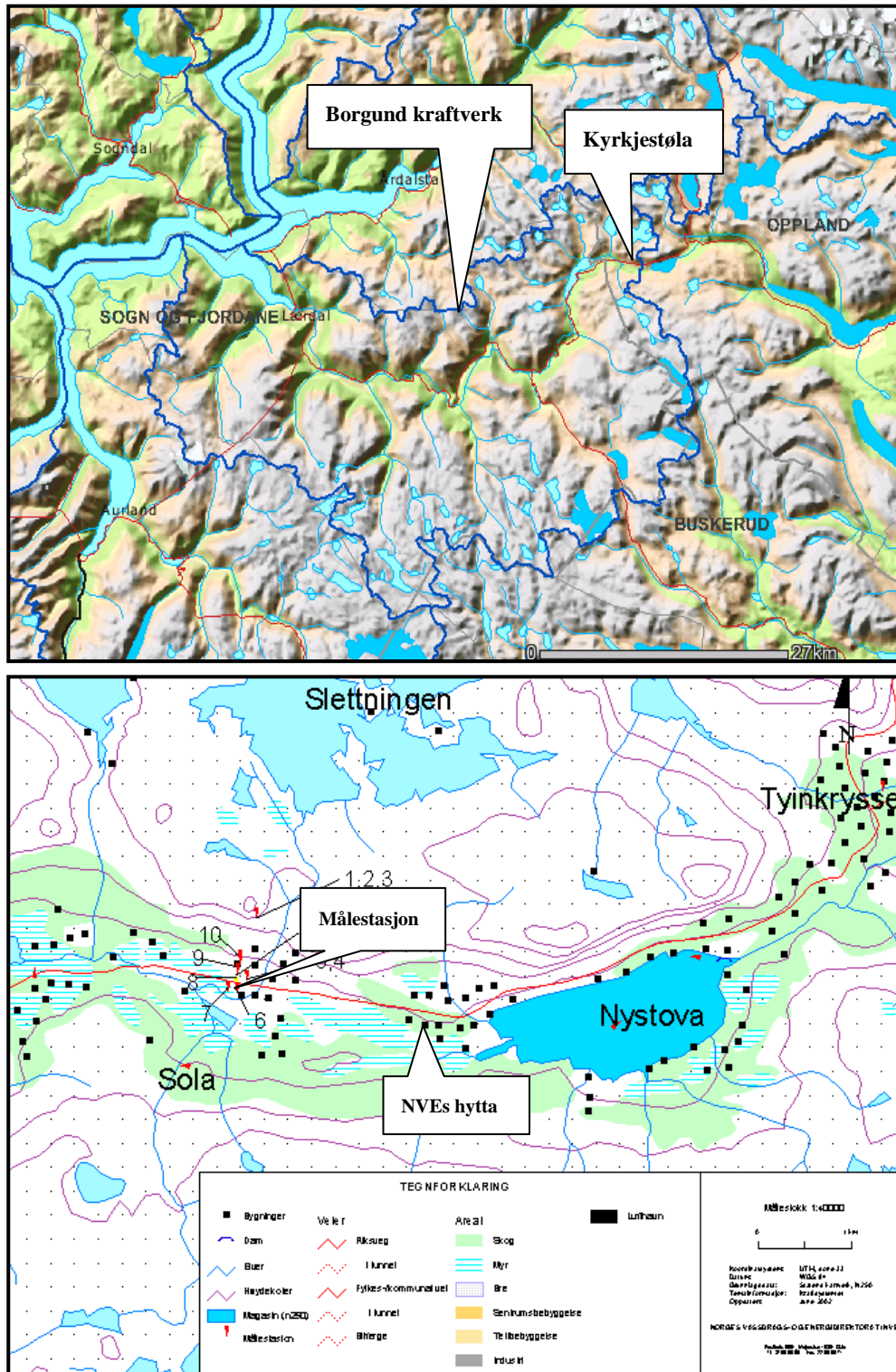
Figur 2. Grunnvannsobservasjoner på Filefjell, Kyrkjestølane.
