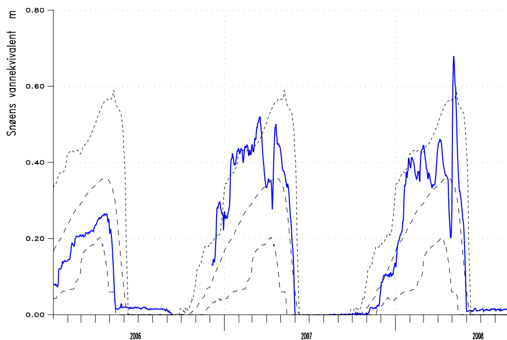
Figur 5. Snøens vannekvivalent målt i 2006-2008 sammenlignet med flereårsmiddel, største og minste observerte snøens vannekvivalent (stiplet) for perioden 1968-1997 (minus årene i perioden 1976-1979, 1989-1993).
