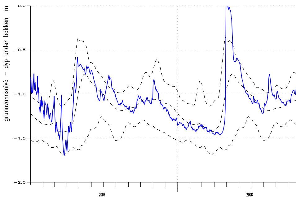
Figur 4. Grunnvannsstand i 2007-2008 (uthevet) sammenlignet med flereårsmiddel største og minste observerte grunnvannsstand (stiplet) 9 , for perioden 1997-2006 i rør-Kyrkjestølane (interpolasjon på 100 dager).
