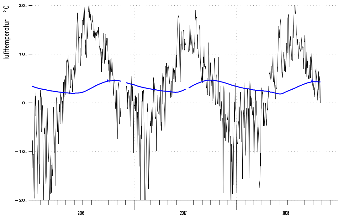
Figur 6. Grunnvann- og lufttemperatur målt i 2006-2008
