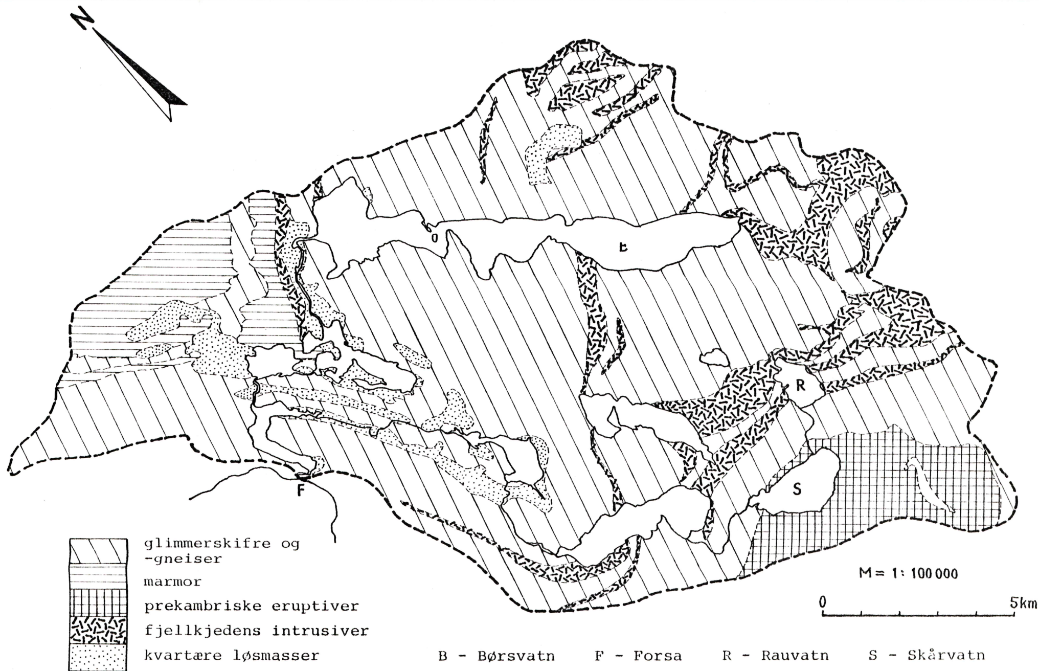
Fig. 4. Forenklet geologisk kart etter Foslie (1941).
