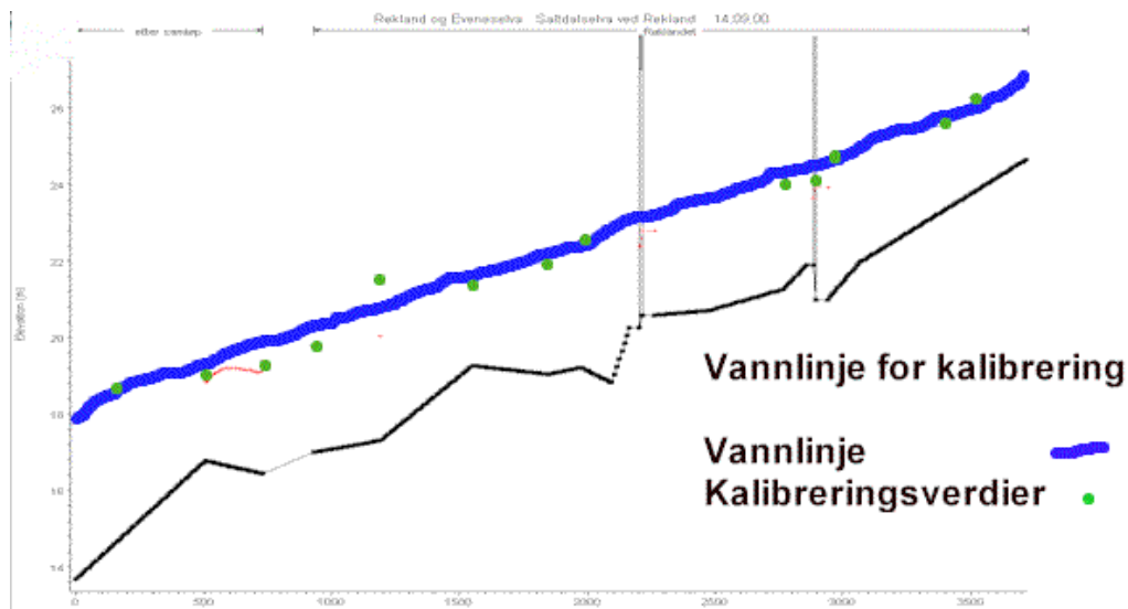
Figur 3-8, lengdeprofil Saltdalselva ved Røkland. Høyeste kalibreringsvannføring med observerte vannstander.
