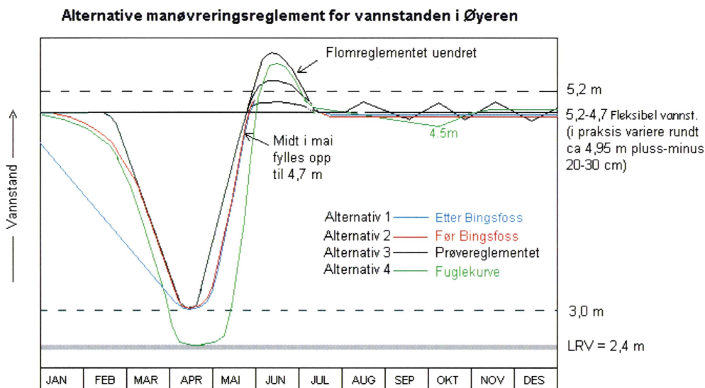
Figur 1.1 Prinsippskisse av de ulike manøvreringsalternativer som har ligget til grunn for de naturfaglige vurderinger. (5,0 m ved Mørkfoss vannmerke tilsvarer kote 101,54 moh).
