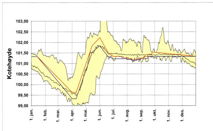
Figur 6.8 Forslag til tidsprofil for vannstand i Øyeren, basert på vannbotaniske kriterier. Målsetningen er å oppnå en median sommervannstand på 101,34 moh (4,80 m). Blå kontrollinje angir en minimums- og rød linje en ønsket maksimumsvannstand. Kurveforløpet utenfor tidsrommet juni-august er ikke like kritisk som for sommerperioden i vegetasjonsmessig henseende. Omhyllingskurven viser høyeste og laveste verdi som er målt i perioden 1978-1999.
