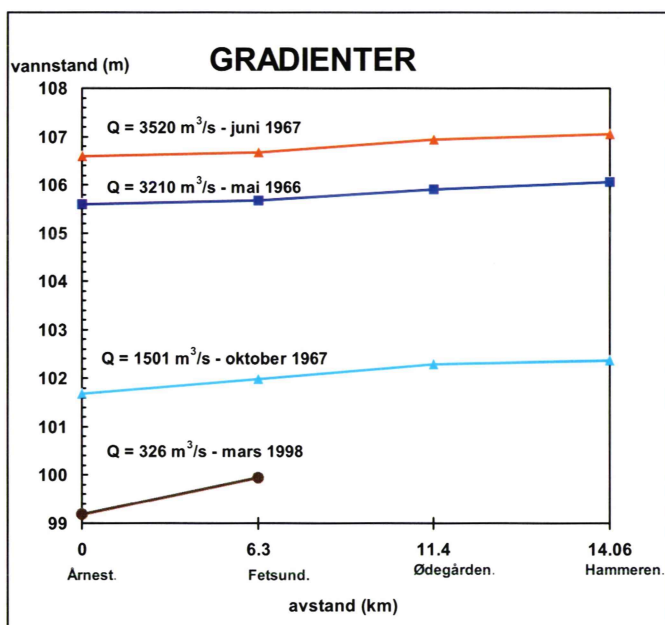
Figur 4.2 Vannlinjer med gradienter i Glomma fra Årnestangen til Hammeren. Vannlinjene er basert på nivellementer av flomvannstander i 1966 og 1967 og vannstandsregistreringer fra 1998. (Data fra NVE).
