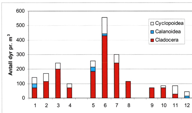
Figur 7.1 Forekomst og dominans av krepsdyr i planktonsamfunnet i Svelle, Snekkervika og i deltaet vest for Svindal i oktober 1994.
